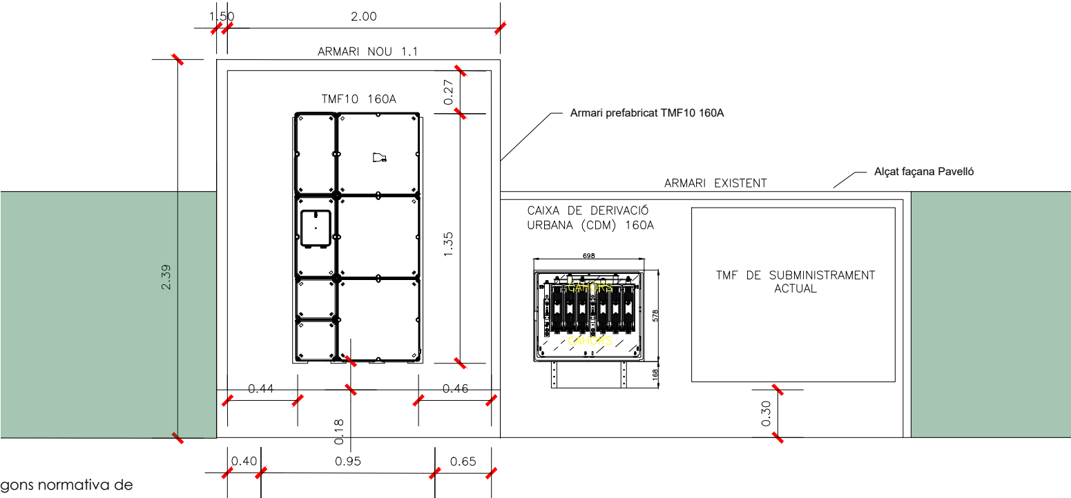
ARMARIS EXTERIORS (E 1:30)
