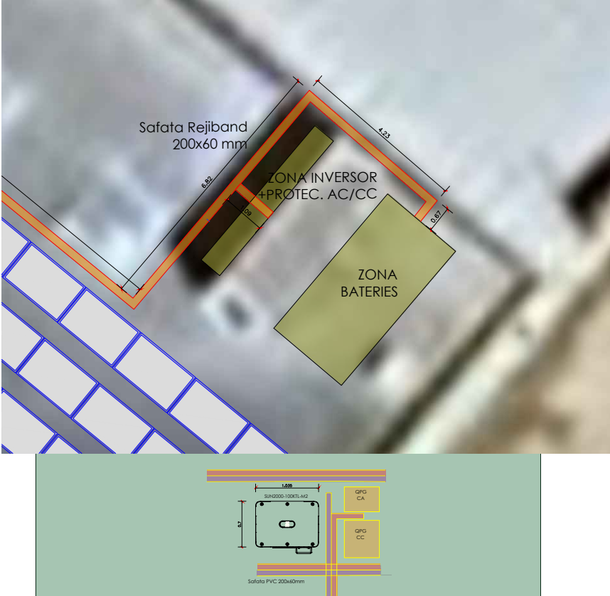
ZONA INVERSOR I PROTECCIONS CA
