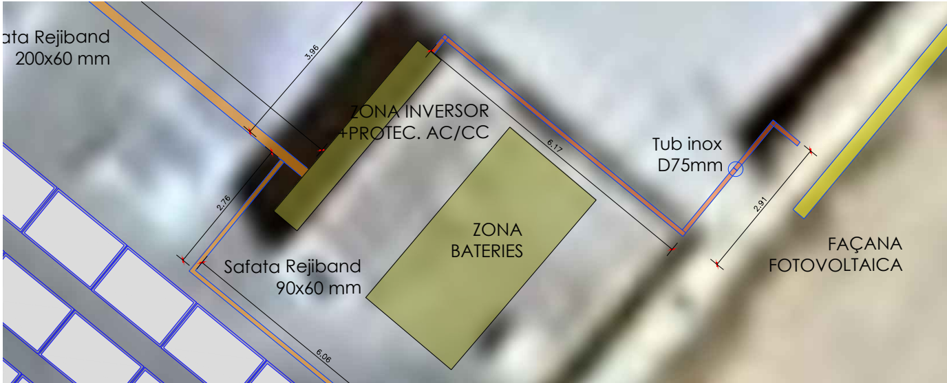
ESQUEMA PAS DEL CABLEJAT DE CORRENT CONTÍNUA - INVERSOR I ARMARIS
