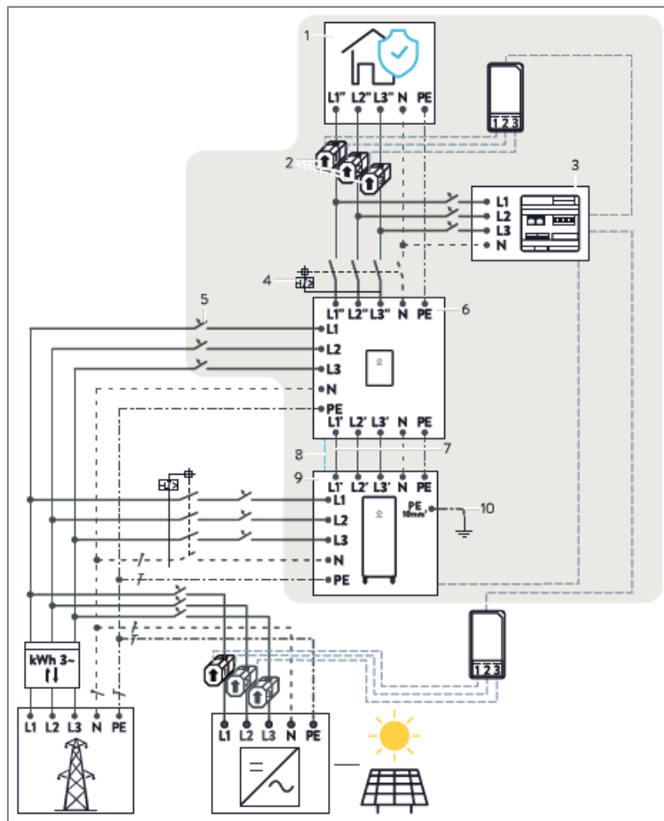
Fig. 21: Esquema sinóptico de connexions: sonnenBatterie 10 performance con sonnenProtect 8000 - Variante de conexión 1
