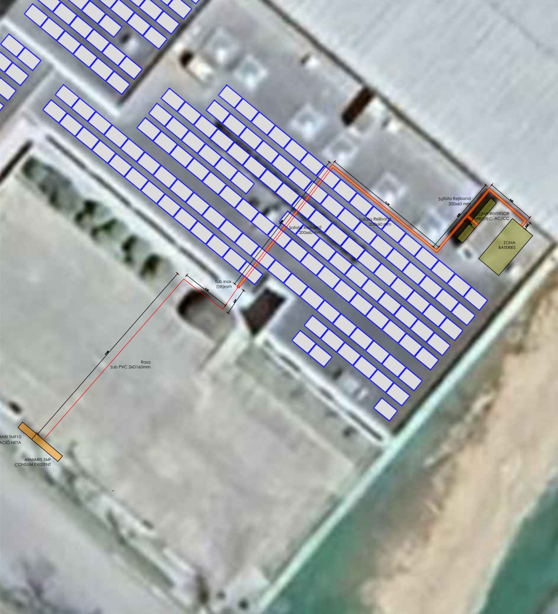
ESQUEMA PAS CABLEJAT CA EXTERIOR
